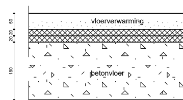
vloer
