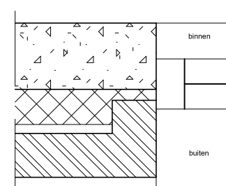
raam
