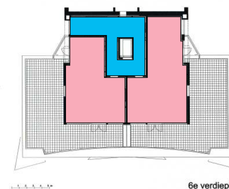
6e verdieping
